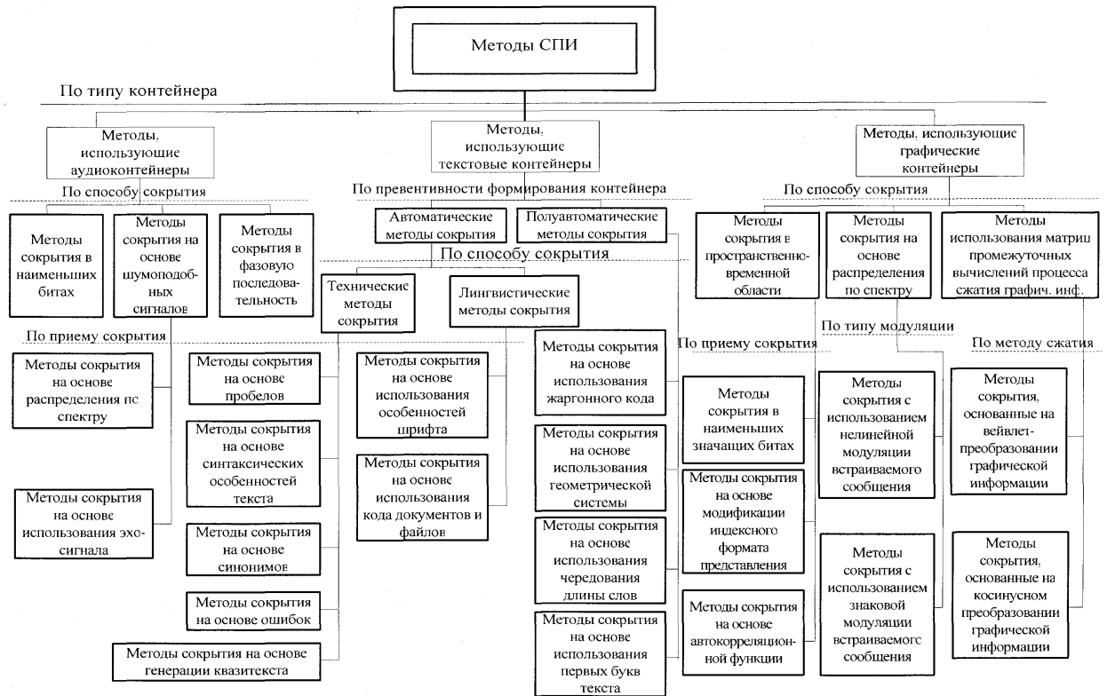
"Рисунок 15. Классификация методов стеганографического преобразования информации (СПИ)"
