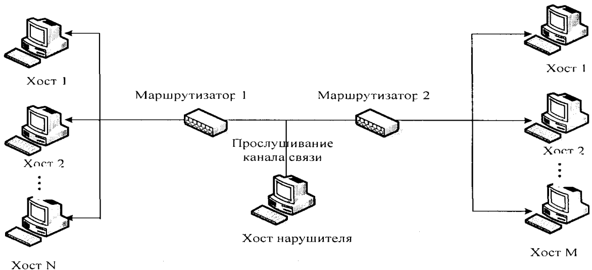
"Рисунок 6. Схема реализации угрозы "Анализ сетевого трафика"
