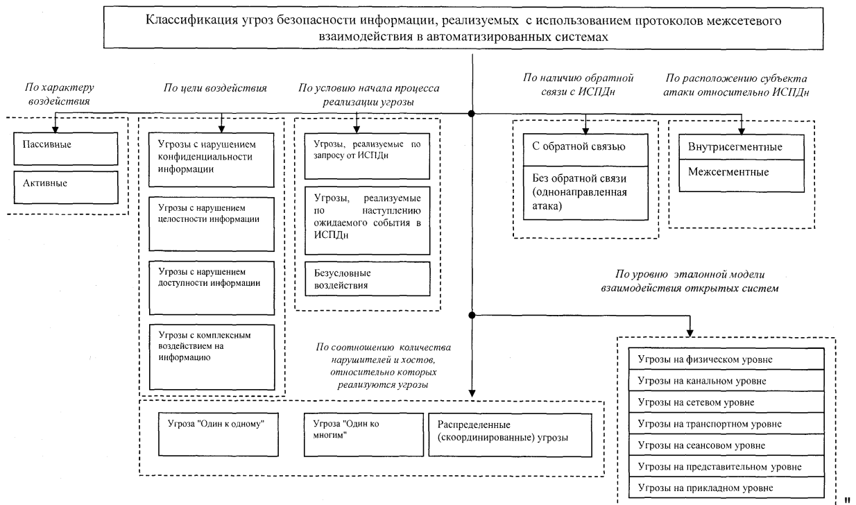
Рисунок 5. Классификационная схема угроз с использованием протоколов межсетевого взаимодействия"
